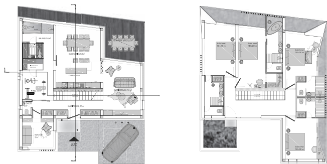
Izgradnja obiteljske Kuće u Jezerima na otoku Murteru
