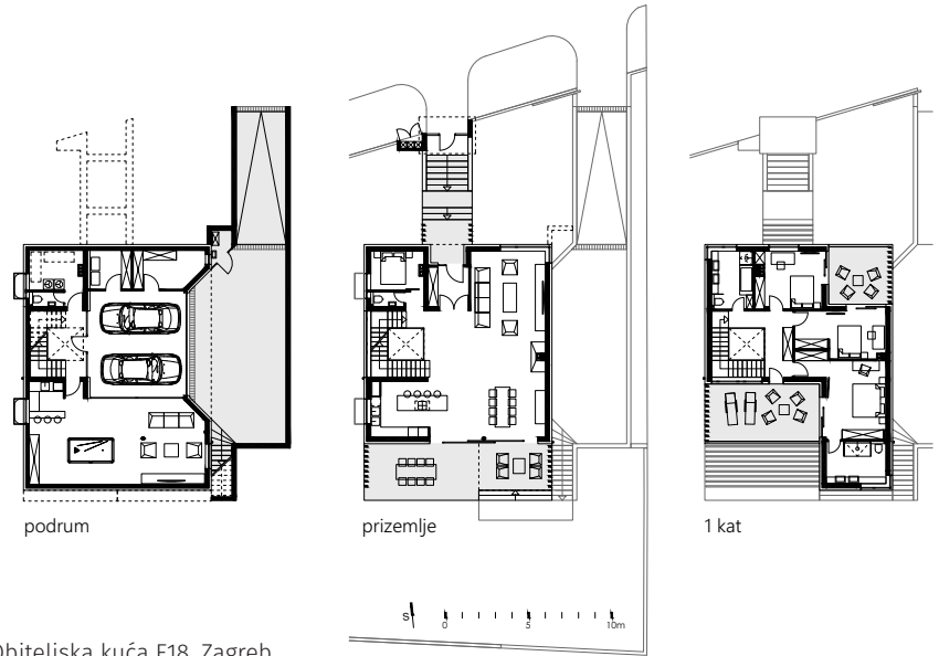
Obiteljska kuća F18, Zagreb
