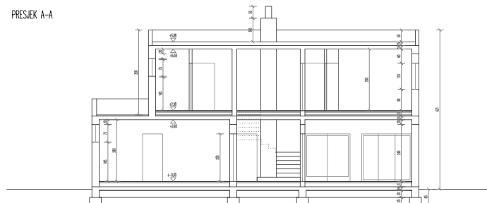
PRESJEK A-A
